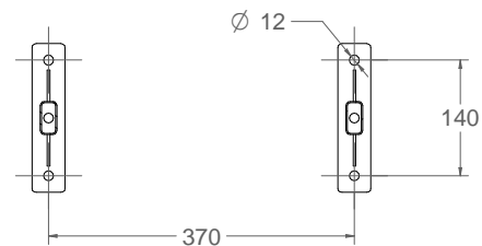
detalle anclaje A-A 1:10
