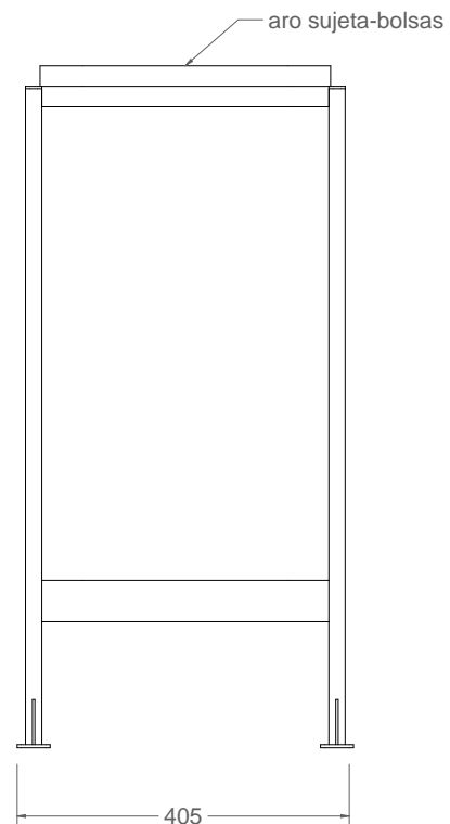
vista alzado 1:10
