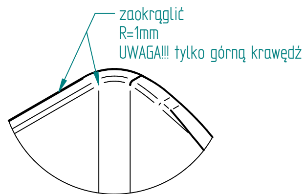
SZCZEGÓŁ A
