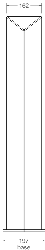
vista alzado 1:10
