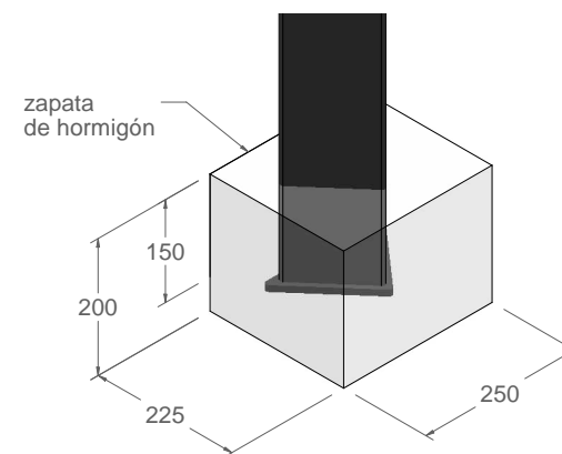
detalle anclaje 1:10
