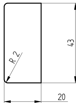
Przekrój deski 1:1
