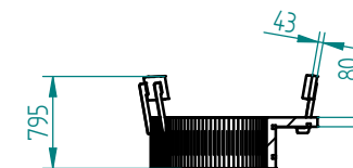
PRZEKRÓJ A-A
