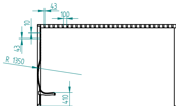
PRZEKRÓJ A-A
